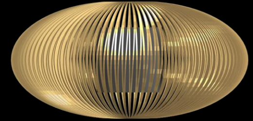
Modell 2072 Pendelleuchte oval Mehrfachgitterstruktur z.B. Messing galvanisiert Mögl. Durchm. 200 – 340 mm 1 x 16 - 24 Watt
